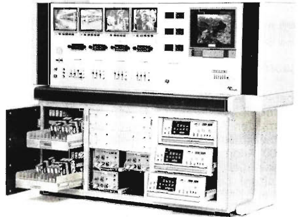
Drei Video-Recorder auf Gleitschienen zum leichten Zugriff (rechts); links der dazugehörige Video-Kassetten-Vorrat auf zwei Archiv-Schüben; in der Mitte das „Kraftwerk“, die vier Leistungsstufen für die Rundfunkprogramme sowie die drei Kabelsender für die eingebauten Video-Recorder Werkfoto
