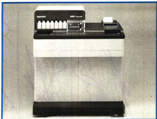
Vollautomatisches Analysensystem mit Methodenprogramm für 16 photometrische Tests und drei ionenselektive Elektrolytbestimmungen Werkfoto
