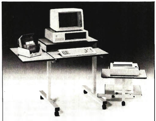
Wif PC-Station für Personal-Computer zur flexiblen Nutzung an verschiedenen Einsatzorten. System 4400 Werkfoto
